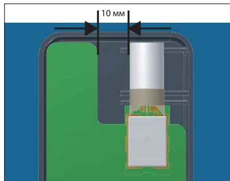
Рис. 20. Внутренний монтаж SL1204/SL1206
