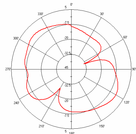
AN1603-868 E-Plane
